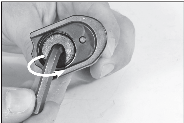
GB Unscrew the bottom of the magazine with the tool provided in the kit. F Dévissez le fond du chargeur à l'aide de l'outil fourni dans la boîte. ES Con la llave de la caja, quitar el tornillo que se encuentra bajo del cargador.
