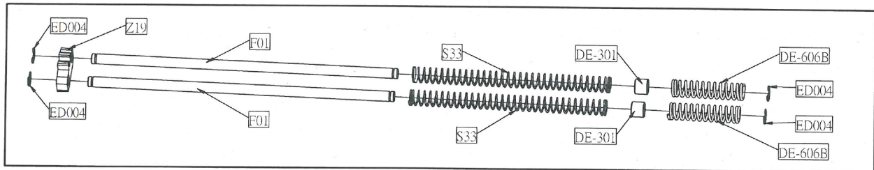
KCCF51-U5 組件
