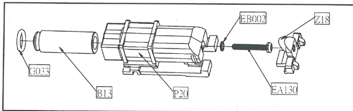
U6 組件
