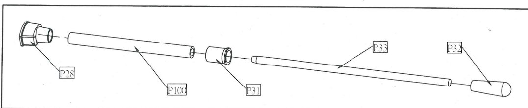
U12 組件
