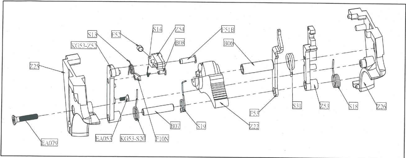
KCCF51-U5 組件
