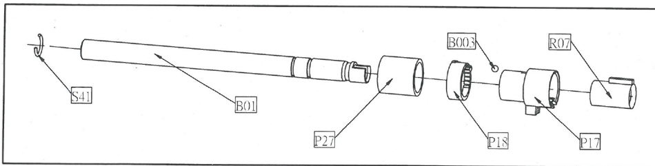
KCCF54-U5 組件
