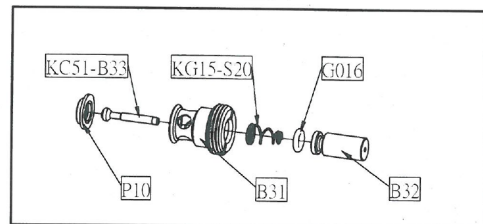
U10 組件
